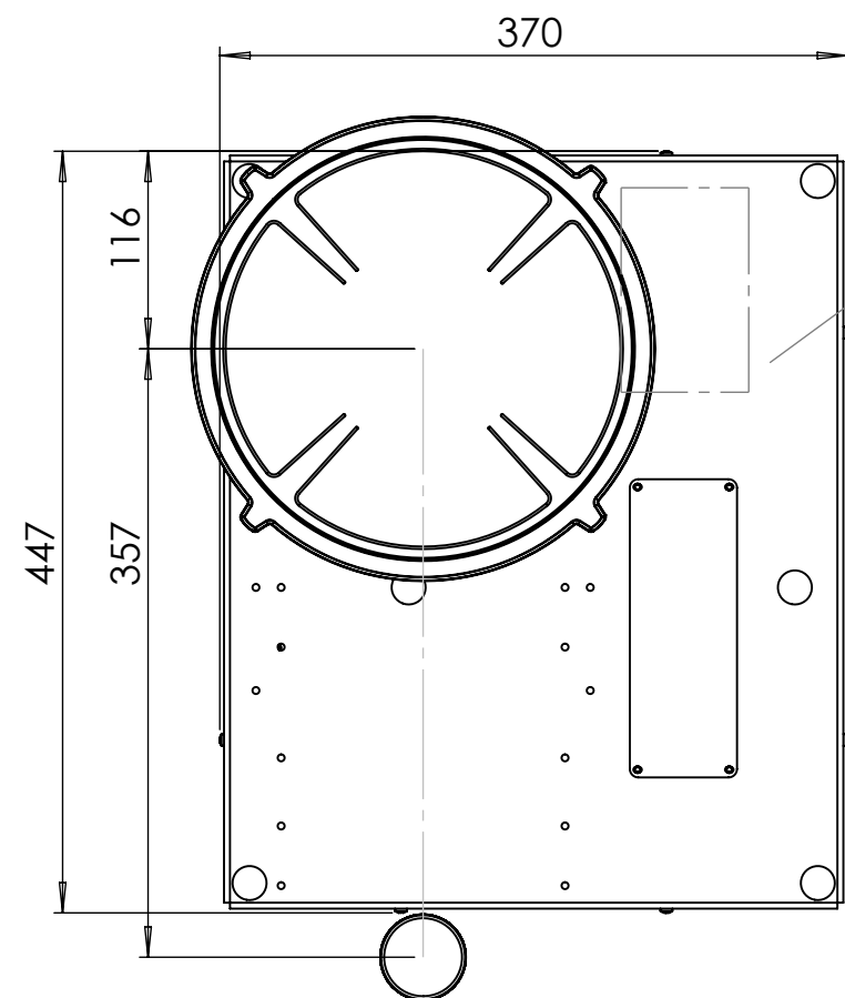
מבט עליון
