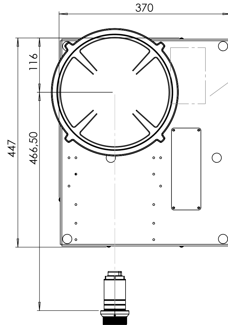
מבט עליון
