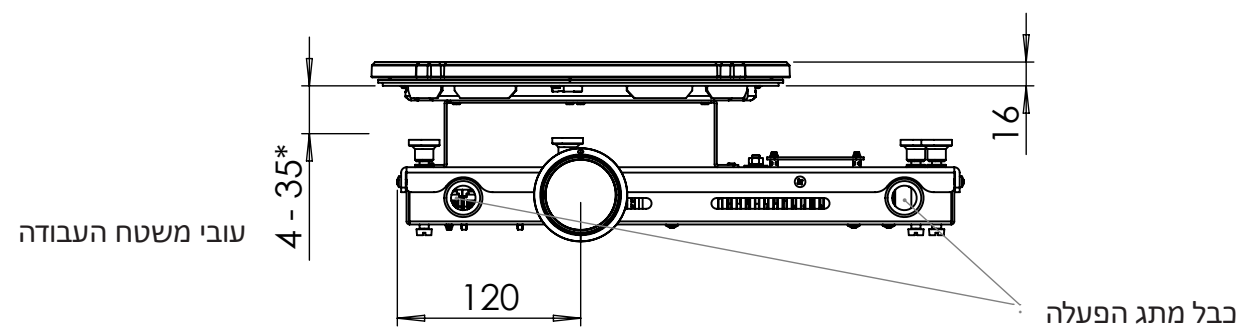
מבט חזיתי
